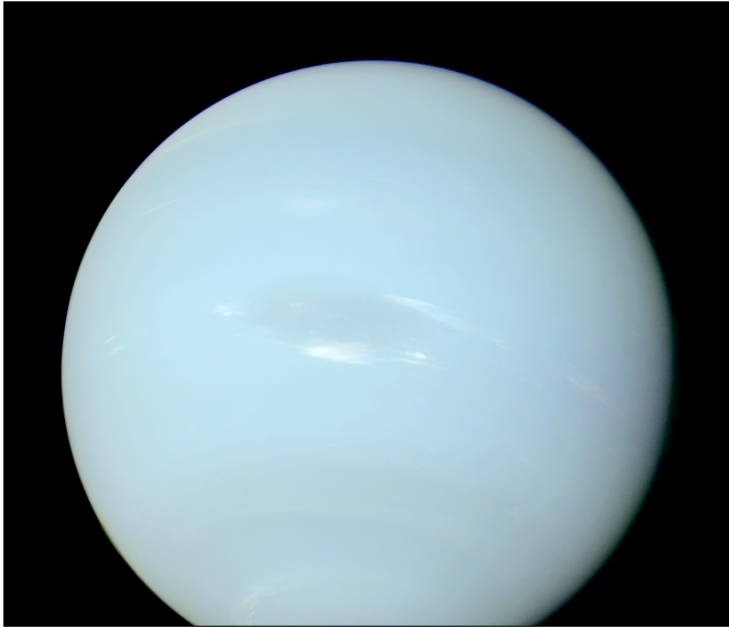
Neptun
