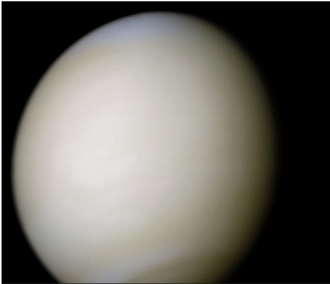
Venus
