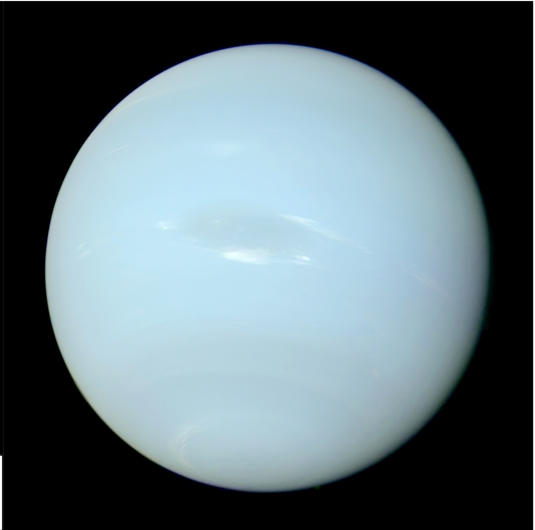
Neptun
