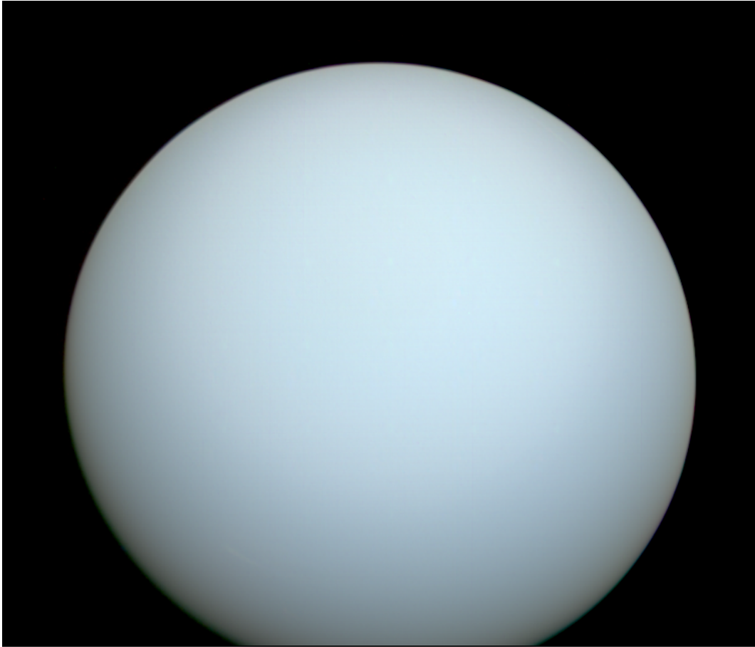
Uran
