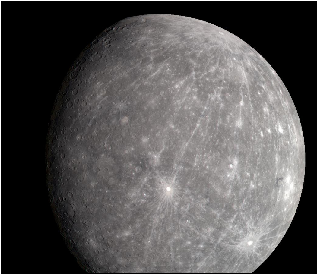
Merkury
