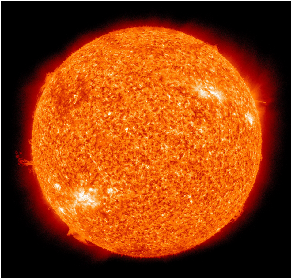
Słońce
