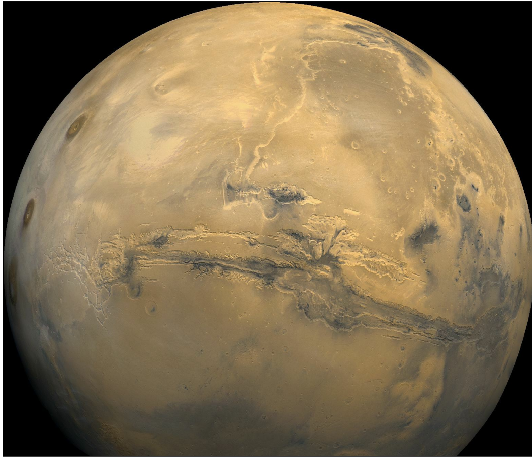
Mars
